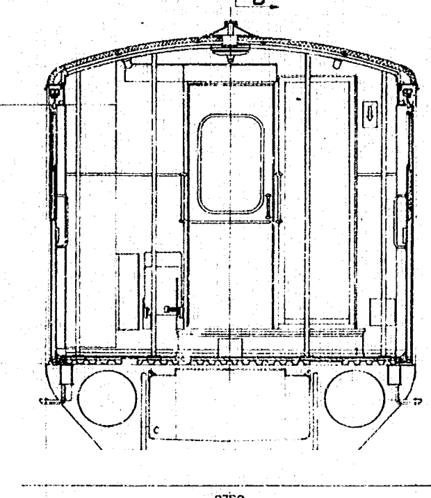
DOORSNEDE B-B
