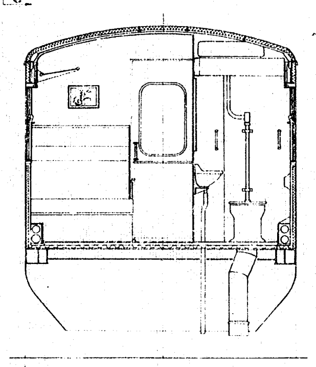
DOORSNEDE C-C
