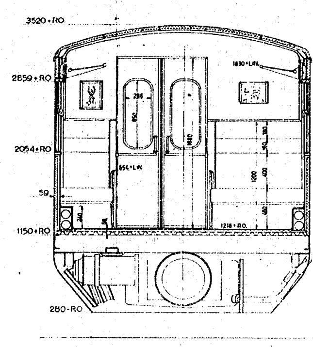
DOORSNEDE A-A
